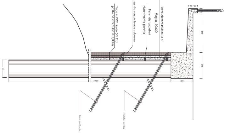
PARETE TIPO C
